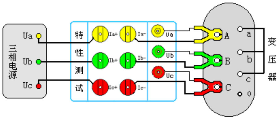
图 7、三相电源测量变压器短路损耗
