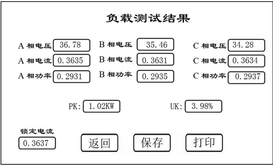
图 9、三相负载测试结果
