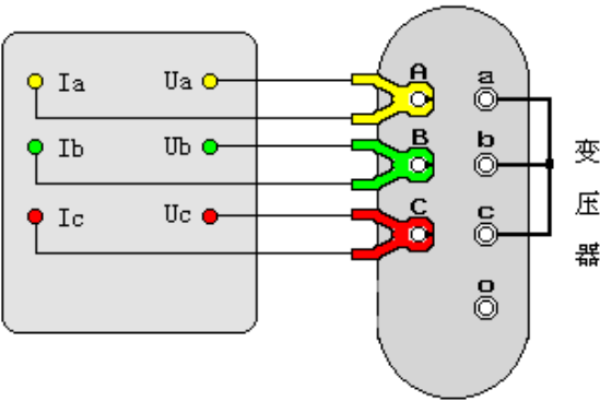
图 3、容量测试接线示意图
